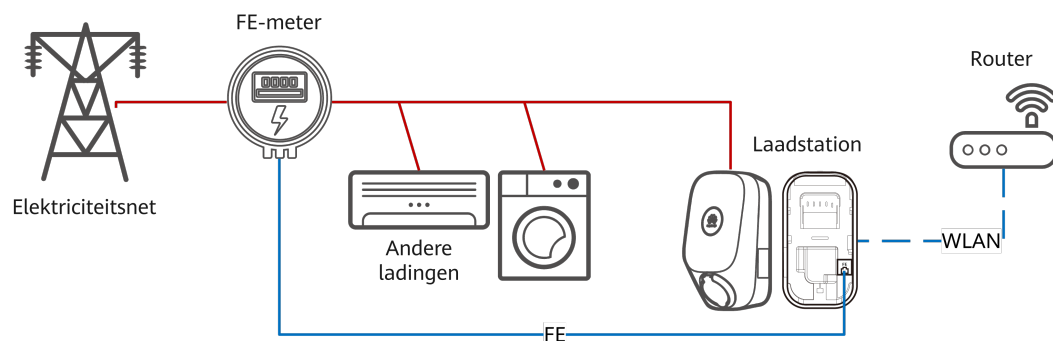
Afbeelding3-1 FE-poort van laadstation direct verbonden met een meter
