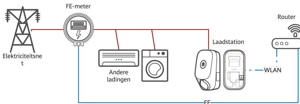
Afbeelding3-3 Laadstation aangesloten op een router via WLAN
